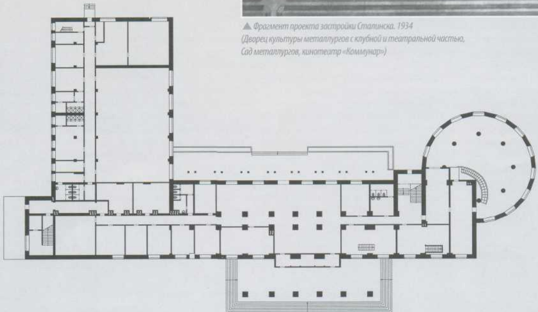
▲ План 1 этажа
