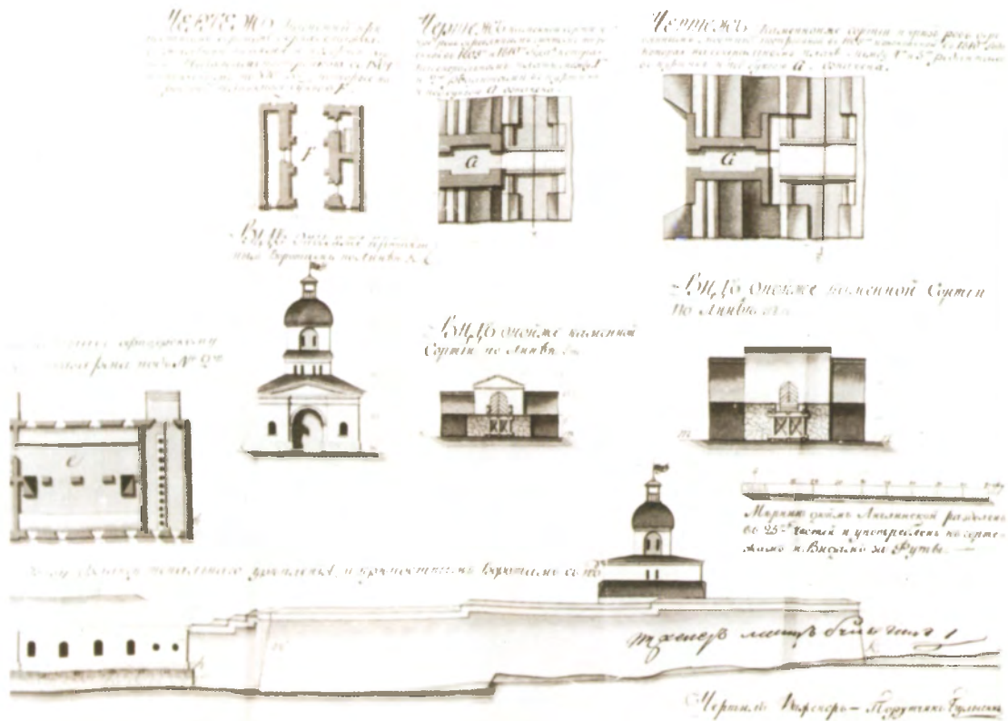
Рис. 4.5. Проектные чертежи крепостных ворот, сортий и надвратной церкви во имя Св. Ильи, выполненные инженер-поручиком Булыгиным. Планы. Фасады. Из фондов РГВИА
