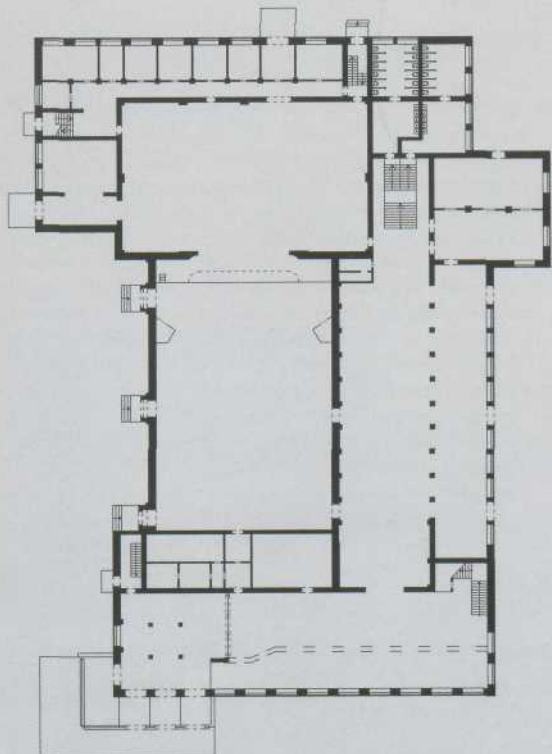
▲ План 1 этажа
